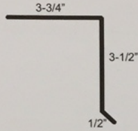
105 Drip Edge
