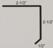
109 2-1/2" Drip Edge
